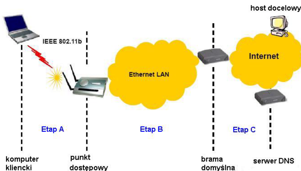
Rys. 31. Etapy komunikacji łączenia klienta z hostem docelowym.
