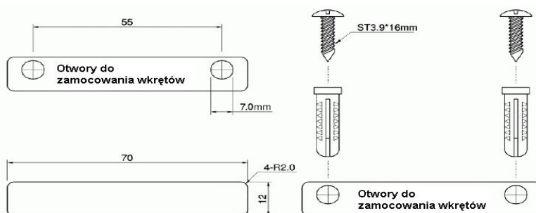
Rys. 1. Montaż urządzenia na ścianie.
